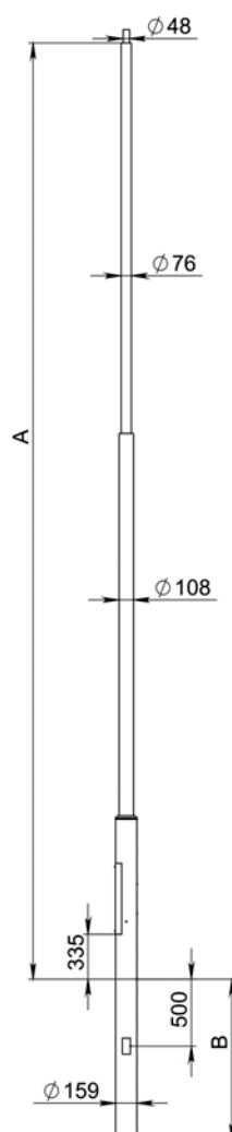
Опора металлическая трубчатая прямостоечная серии МНТ-П-Х/Х-02-Х
